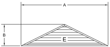
Pyramid (E)
