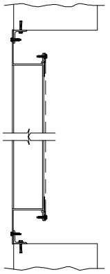
ANGLE SUBFRAME
